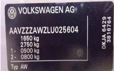
VIN PLATE OR STICKER
